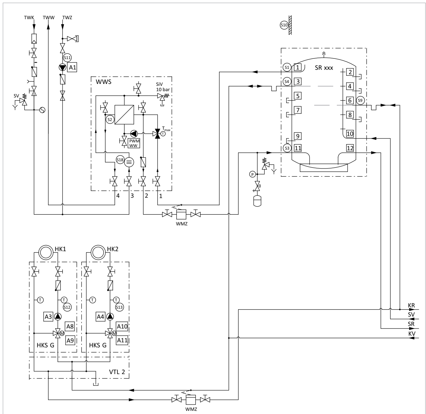
Abb. 5: SolvisDirekt 3 mit Pelletkessel SolvisLino 4, Solar und Festbrennstoffkessel, ohne Zirkulationsentkopplung – Teil 1
