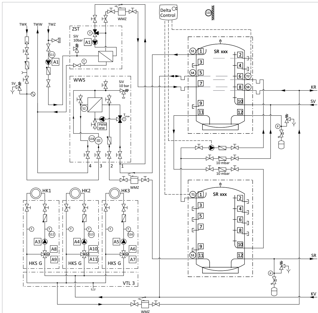
Abb. 13: SolvisDirekt 3 mit Zirkulationsentkopplung, Erweiterungsspeicher und Solaranbindung – Teil 1
