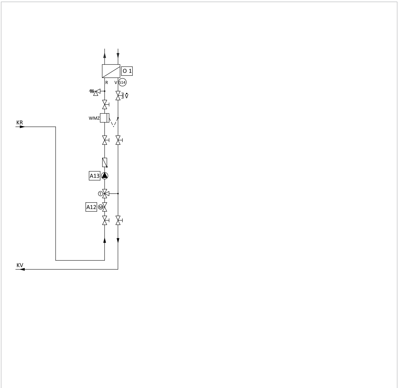
Abb. 18: SolvisDirekt 3 mit Zirkulationsentkopplung – Teil 2
