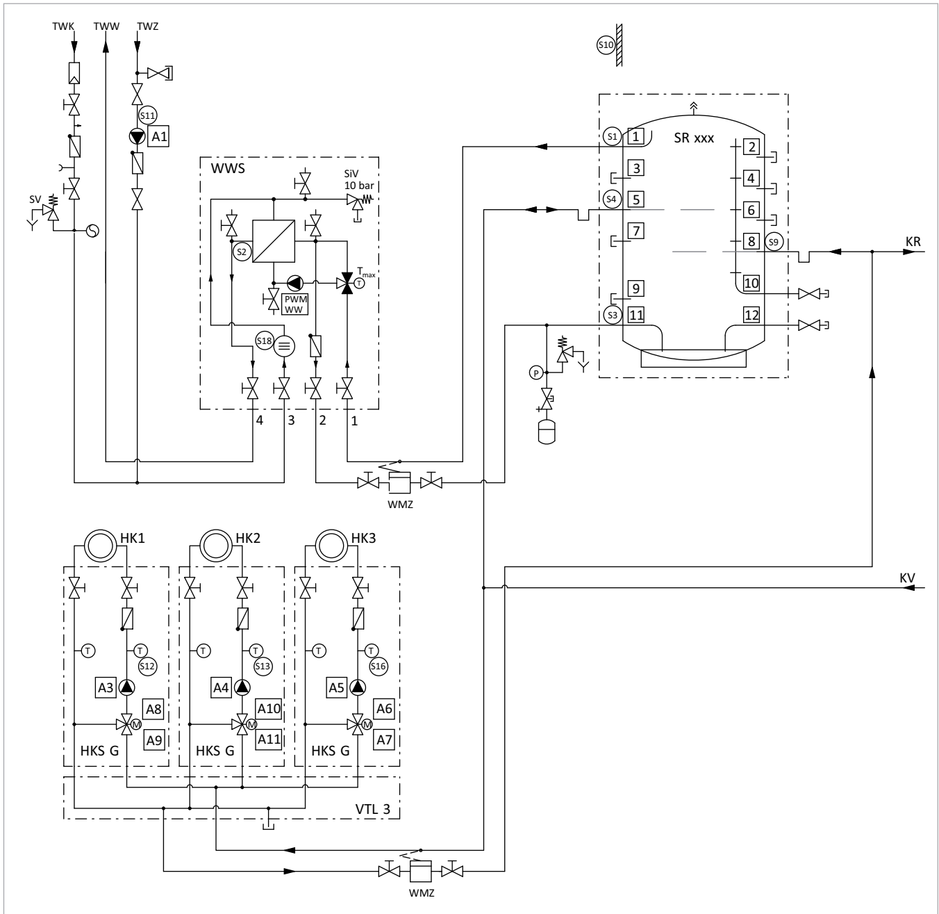
Abb. 7: SolvisDirekt 3 ohne Zirkulationsentkopplung – Teil 1
